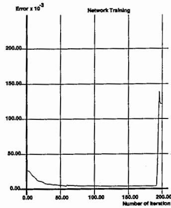
図 7: 学習の様子 (入力セット数: 5, 中間ユニット数: 17)
