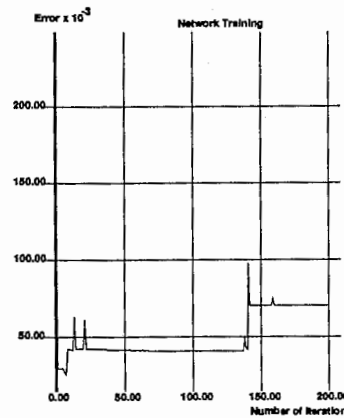
図 9: 学習の様子 (入力セット数: 5, 中間ユニット数: 68)
