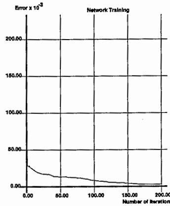
図 8: 学習の様子 (入力セット数: 5, 中間ユニット数: 34)
