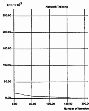
図 16: 学習の様子 (中間ユニット数 : 25)
