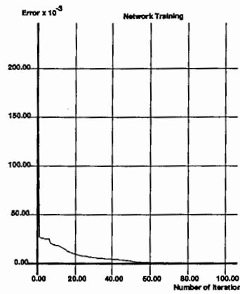
図 4: 学習の様子 (入力セット数 : 3, 中間ユニット数 : 17)
