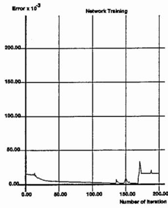
図 14: 学習の様子 (中間ユニット数 : 9)
