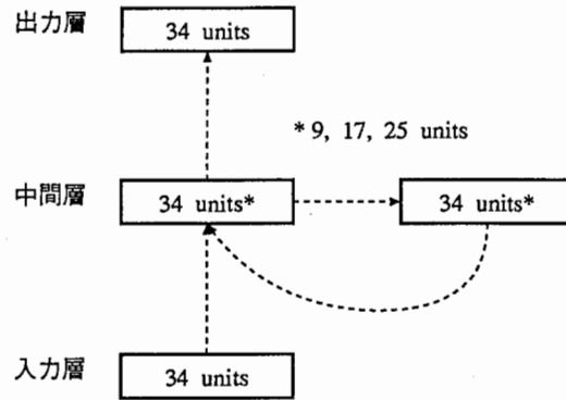
図 13: リカレント型ネットワークの構造
