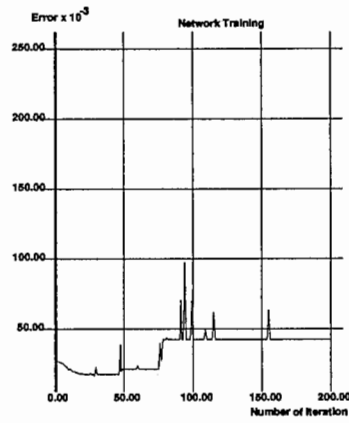
図 11: 学習の様子 (入力セット数 : 7, 中間ユニット数 : 34)
