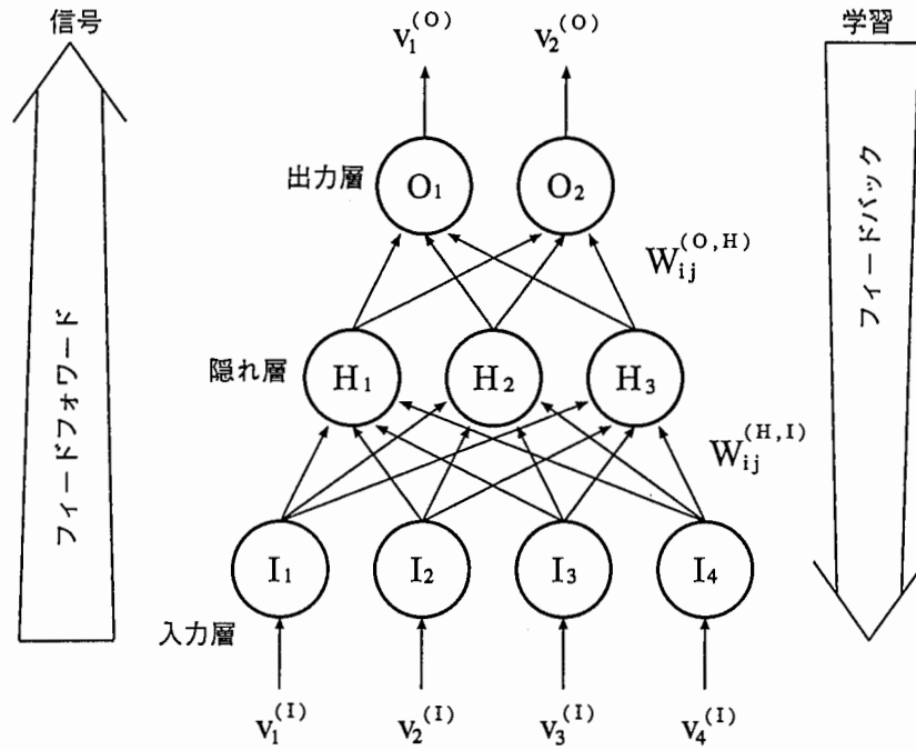
図 2: 階層型モデル (バックプロパゲーションモデル)
