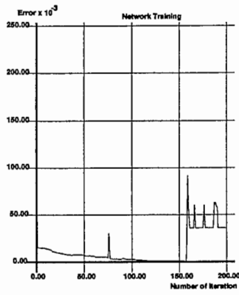
図 15: 学習の様子 (中間ユニット数 : 17)
