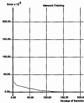
図 5: 学習の様子 (入力セット数 : 3, 中間ユニット数 : 34)
