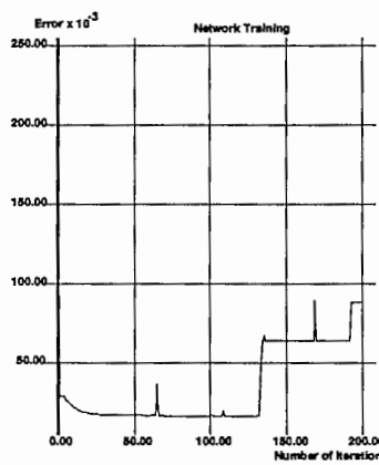
図 6: 学習の様子 (入力セット数 : 3, 中間ユニット数 : 68)
