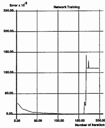
図 10: 学習の様子 (入力セット数 : 7, 中間ユニット数 : 17)
