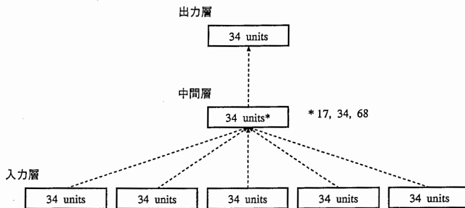
図 3: フィードフォワード型ネットワークの構造
